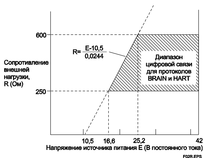
Рис. 2. Взаимосвязь между напряжением источника питания и сопротивлением внешней нагрузки (Коды выходного сигнала D и J)
